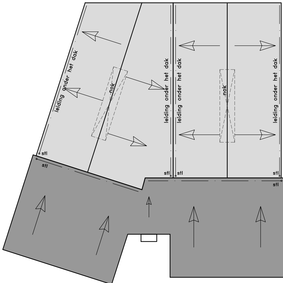
Dakoverzicht / hemelwateroverzicht * afm. en plaats noodoverlopen volgens opgave constructeur * afschot 16mm/m — riolering o stl standleiding vacuümsysteem (pluvia o.g.) o hwp hemelwater verzamelpunt vacuümsysteem (pluvia o.g.) conform opgave constructeur
